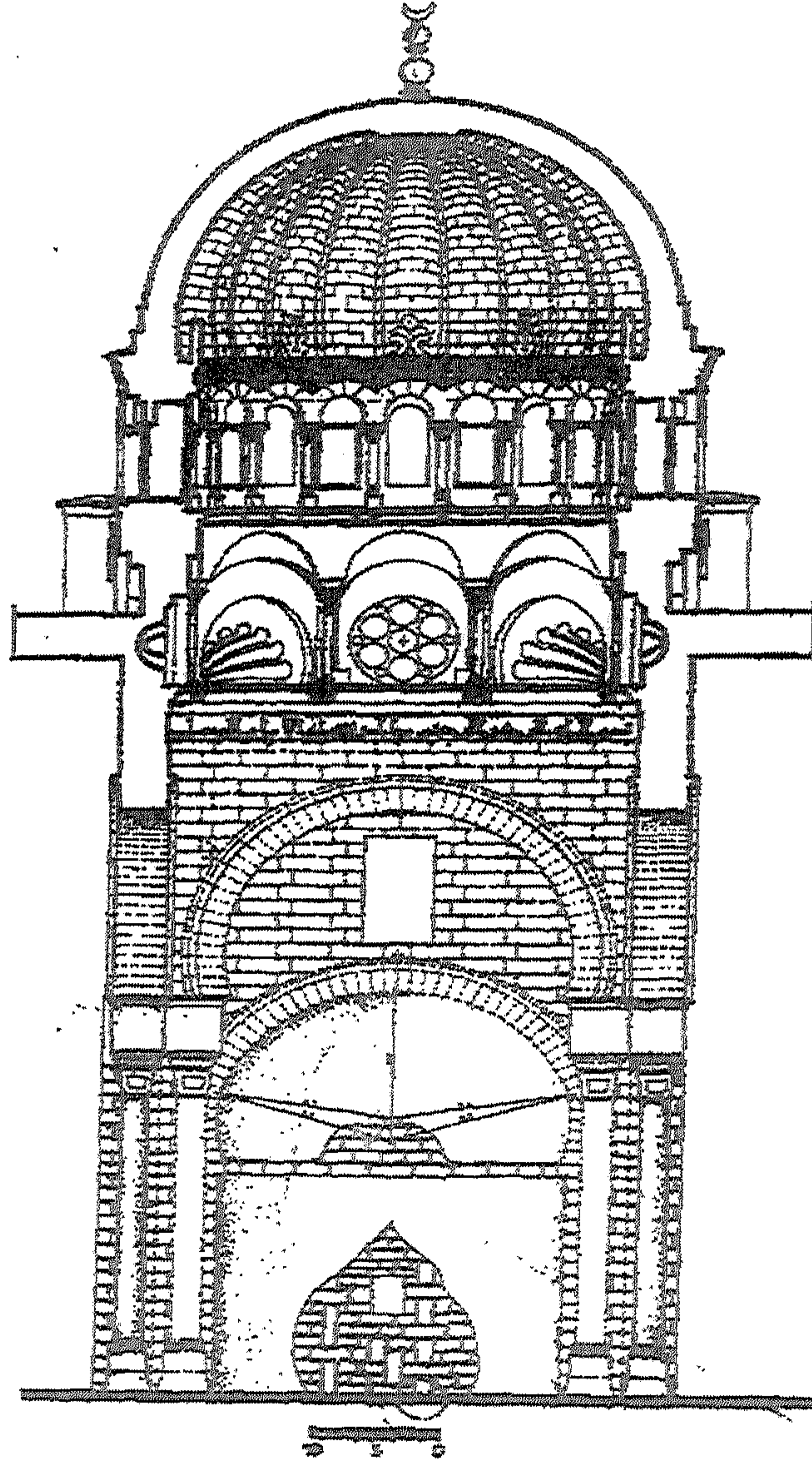
(شكل رقم ٧١) مقطع عمودي على قبة المحراب بجامع الزيتونة عن د/ الدولاتلي.
